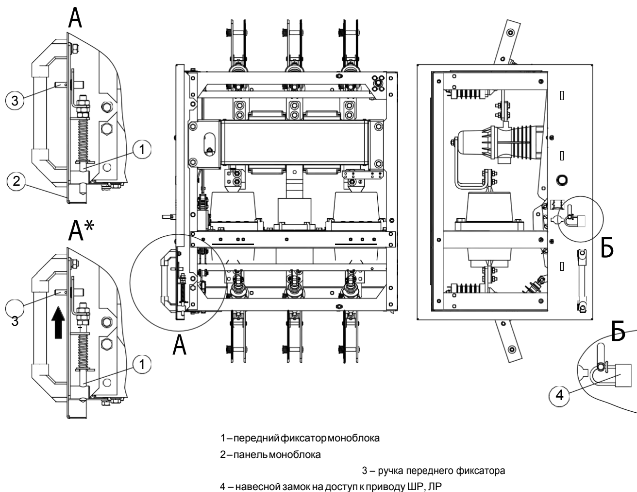
Рис. 5.7. Общий вид моноблока
