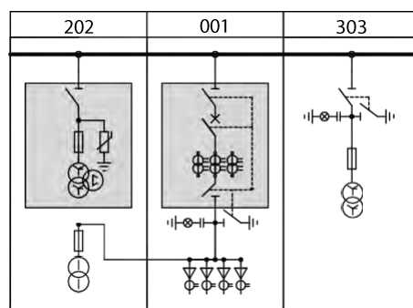
Рис. 8.2.2. Однолинейная схема первого включения ВВ
