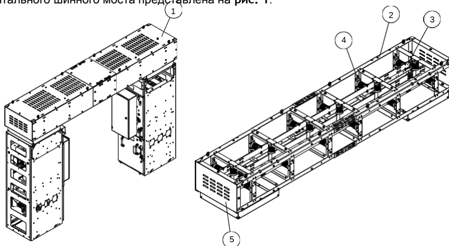
1- Верхний защитный экран; 2- Металлоконструкции; 3- ошинока; 4- опорные изоляторы; 5- Боковые защитные экраны
