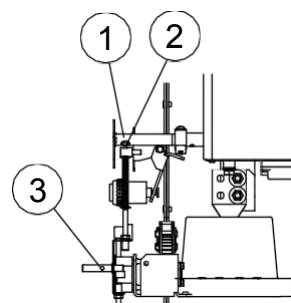
Рис. 9.2. Система блокировок камеры КСО «Новация»
