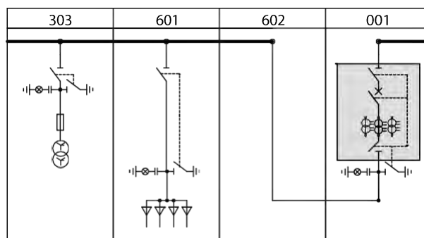
Рис. 8.1. Однолинейная схема кабельного ввода
