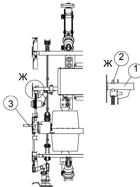
Рис. 9.1. Система блокировок камеры КСО «Новация»
