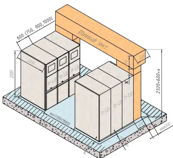
Рис. 1.19. Шинный мост секционирования с боковыми приставками
