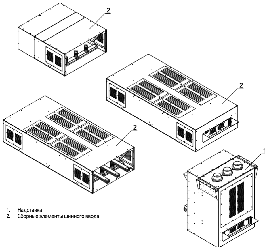
Рис. П7.3. Составные сборочные элементы конструкции шинного ввода
