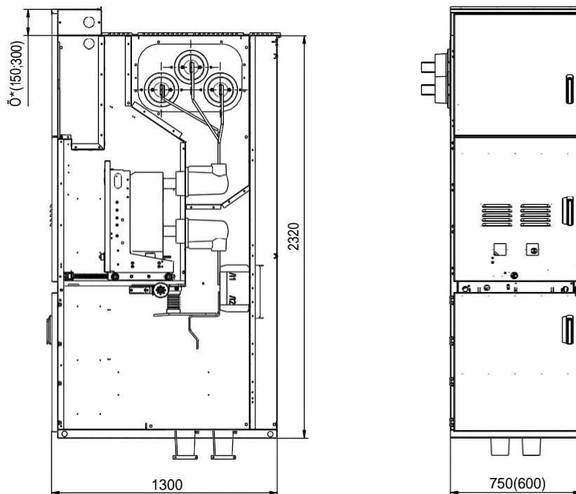
Рис. ПЗ.1. Шкаф КРУ D-12P с силовым выключателем на номинальный ток до 2000 А
