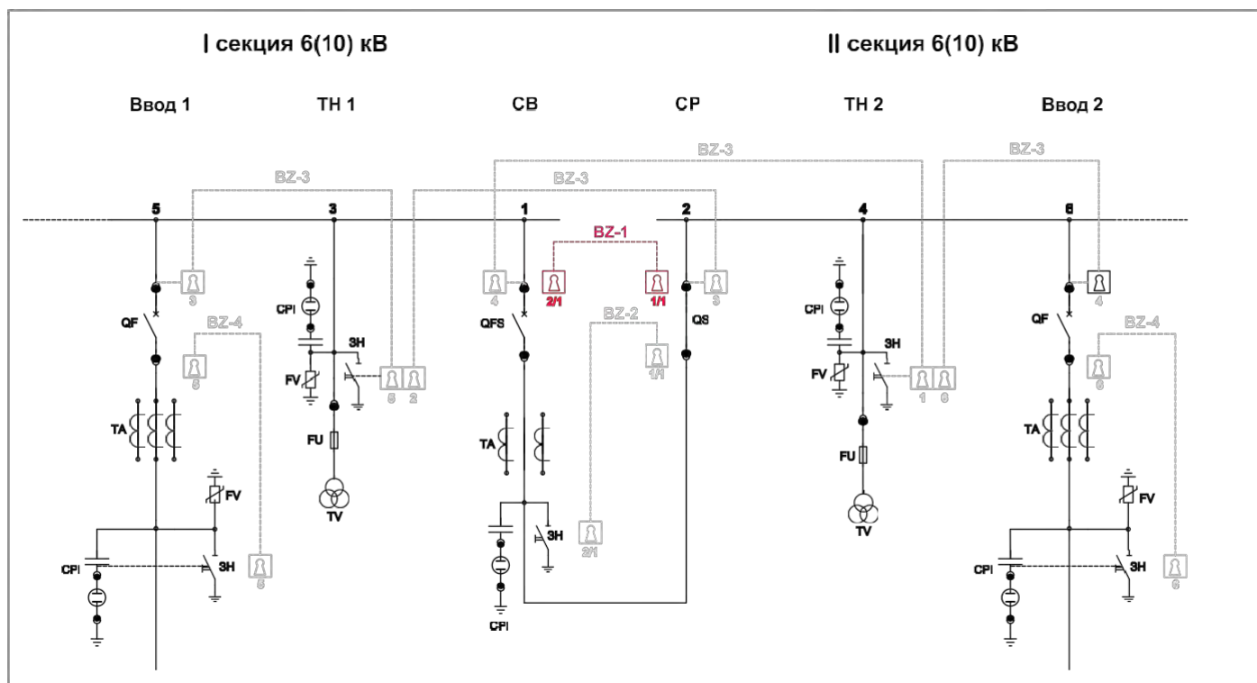
Рис. 1.43. Поясняющая схема размещения замковых блокировок BZ-1
