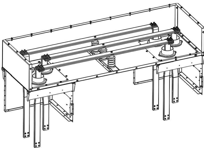
Рис. П7.9. Соединение шин внутри шинного моста
