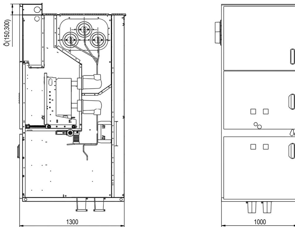
Рис. ПЗ.3. Шкаф КРУ D-12P с силовым выключателем на номинальный ток до 3150 А
