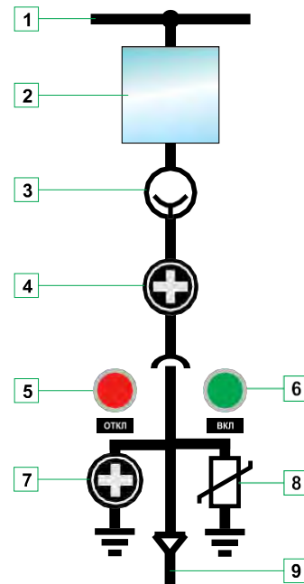
Рис. 1.47. Пример базовой мнемосхемы шкафа ввода/ОЛ
