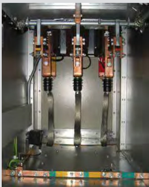
Рис.1.11. Отсек присоединений
