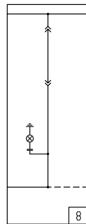
8 Шкаф секционного разъединителя Ввод/вывод шинами вбок
