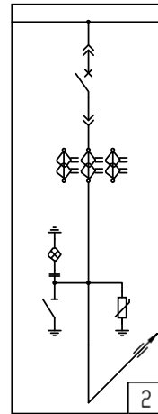
2 Шкаф с силовым выключателем Ввод/вывод шинами сзади
