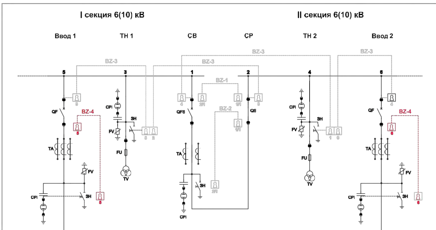
Рис. 1.46. Поясняющая схема размещения замковых блокировок BZ-3
