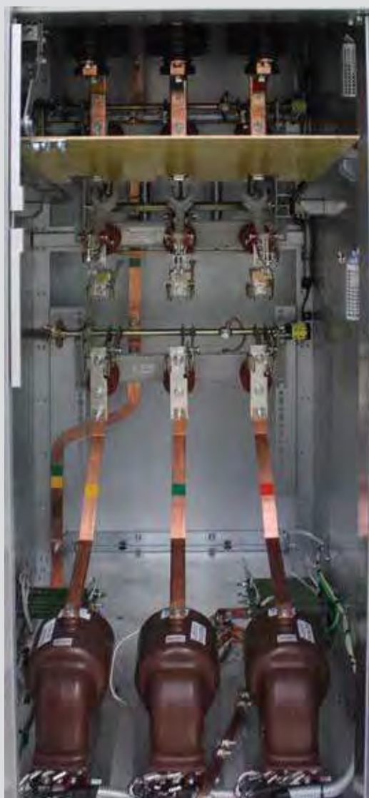
Рис 1.35. Выключатель нагрузки в шкафу со стационарно размещенным ТН
