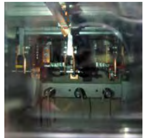
Рис. 2.11. Вид на контакты заземлителя через смотровое окно отсека
