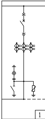
1 Шкаф с силовым выключателем Ввод/вывод шинами сбоку
