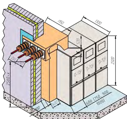
Рис. 1.17. Шинный ввод сбоку с боковой приставкой
