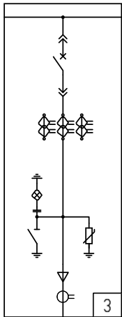
3 Шкаф с силовым выключателем Ввод/вывод кабелем снизу
