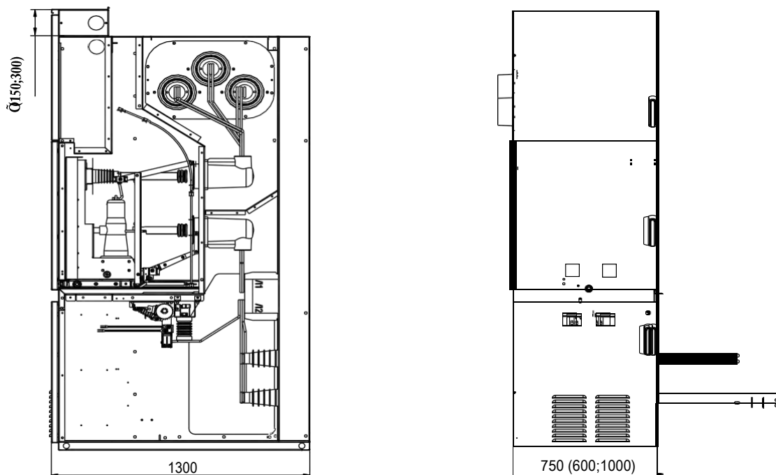
Рис. ПЗ.5. Шкаф КРУ D-12P с секционным выключателем
