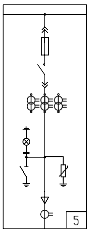
5 Шкаф с контактором Ввод/вывод кабелем снизу
