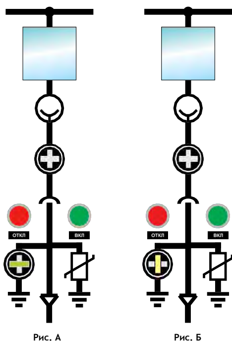
Рис. 1.49. Состояние мнемосхемы при нахождении КВЭ в разобщенном положении
