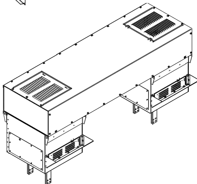
Рис. П7.10. Шинный мост в сборе
