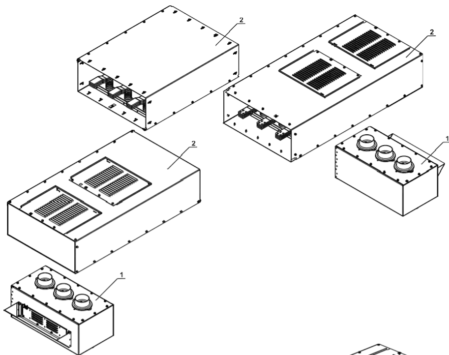
Рис. П7.5. Составные сборочные элементы конструкции шинного моста
