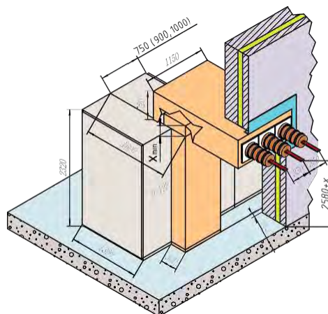
Рис. 1.18. Шинный ввод сзади с задней приставкой (X min = 200 мм)
