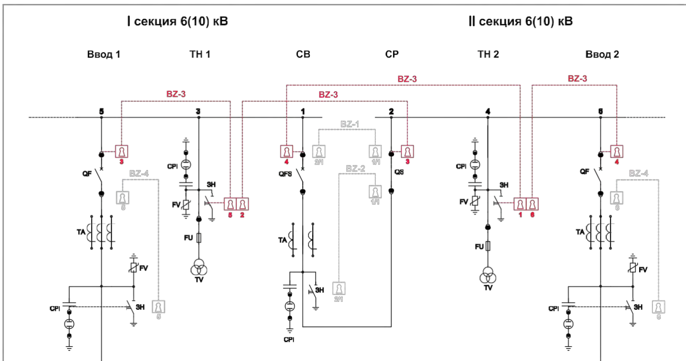
Рис. 1.45. Поясняющая схема размещения замковых блокировок BZ-3
