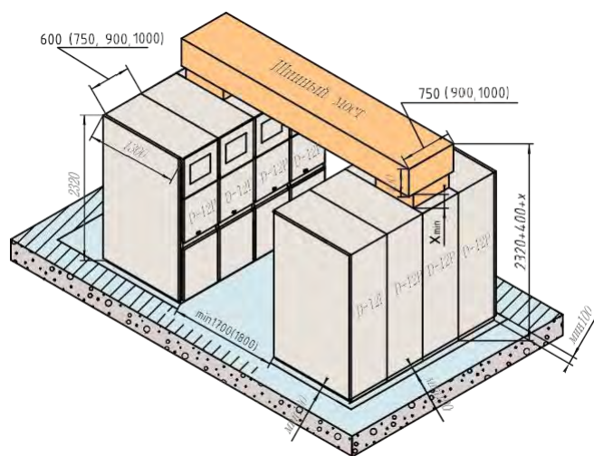
Рис. 1.21. Шинный мост систем сборных шин секций (X min = 200 мм)
