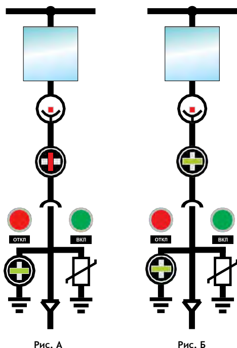
Рис. 1.50. Состояние мнемосхемы при нахождении КВЭ в рабочем положении
