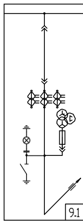
Шкаф с разъединителем и измерительным тр-ром Ввод/вывод шинами сзади
