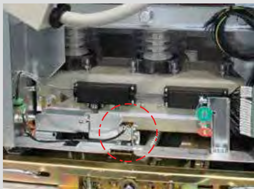
Рис. 2.39. Расположение блокировки Y0 в шкафу с выключателем ВВ/ТЕЛ типа ISM15_LD
