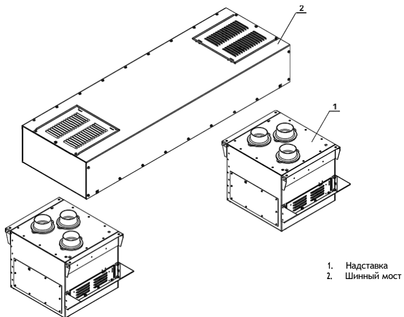
Рис. П7.8. Составные сборочные элементы конструкции шинного ввода
