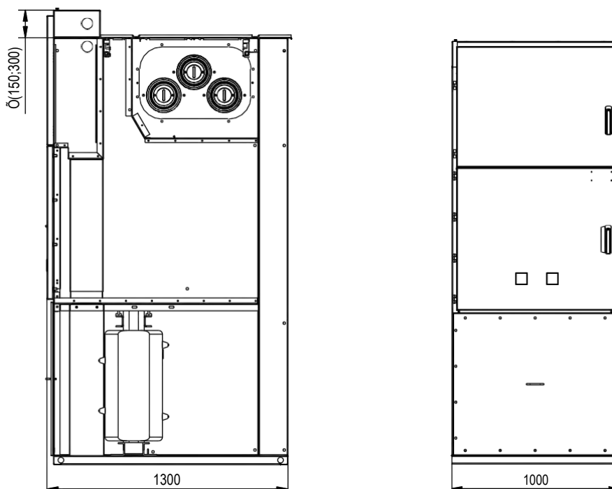
Рис. ПЗ.10. Шкаф ТСН мощностью 63 или 100 кВА
