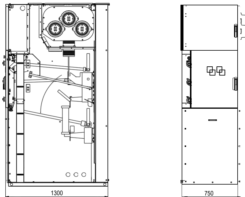
Рис. ПЗ.9. Шкаф организации питания ТСН (вариант с подключением на сборные шины)
