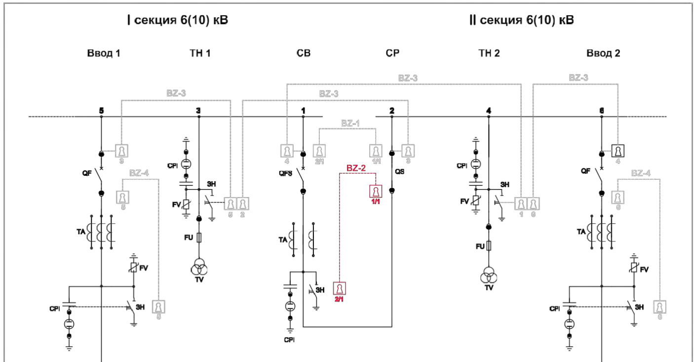
Рис. 1.44. Поясняющая схема размещения замковых блокировок BZ-2
