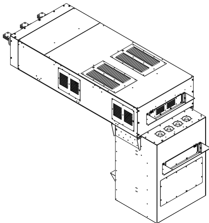
Рис. П7.2. Шинный ввод в сборе
