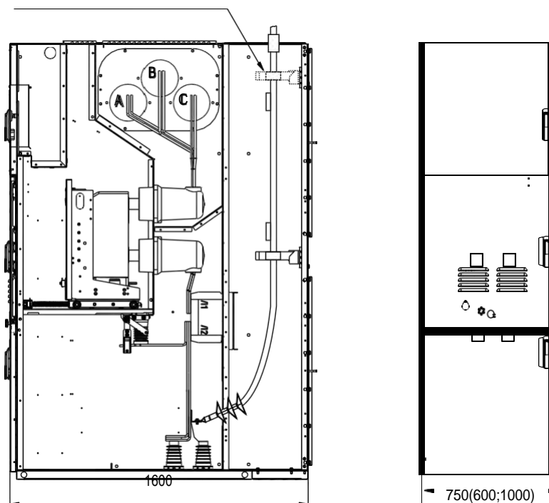
Рис. ПЗ.12. Шкаф КРУ D-12P с подключением кабеля сверху через заднюю шинную приставку
