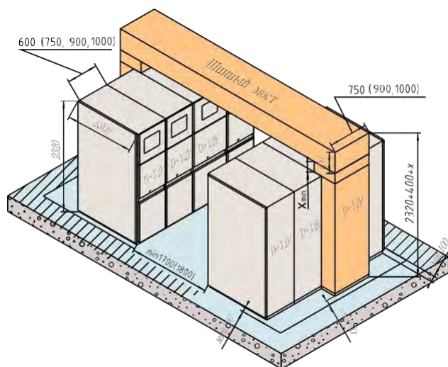
Рис. 1.20. Шинный мост секционирования с задними приставками (X min = 300 мм)
