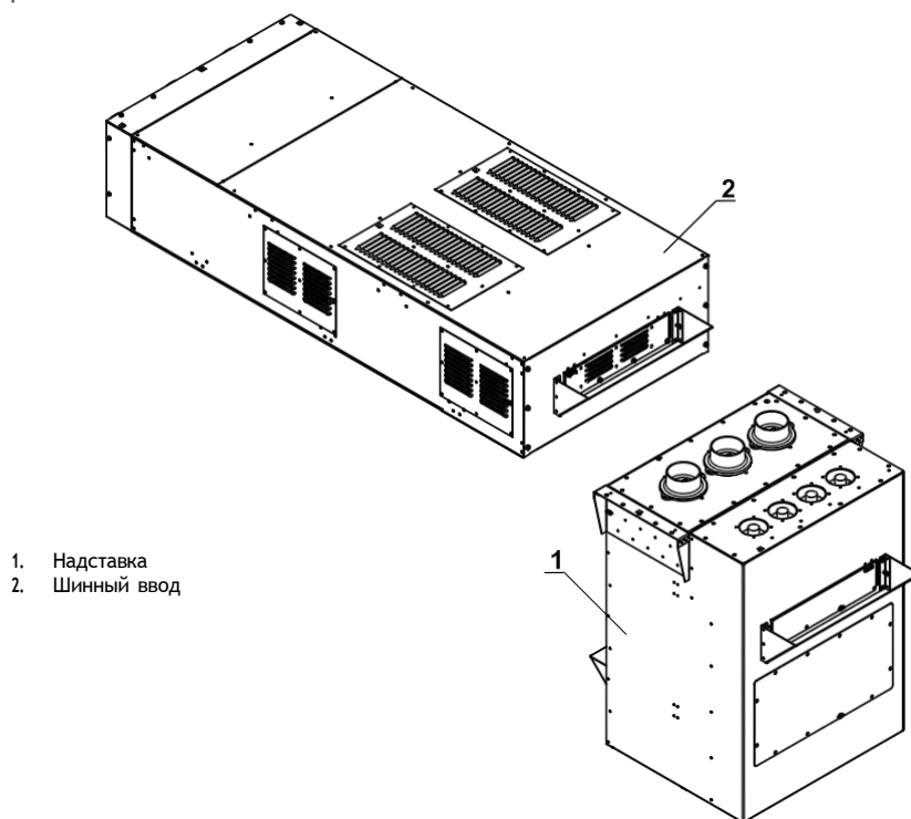
Рис. П7.1. Составные сборочные элементы конструкции шинного ввода
