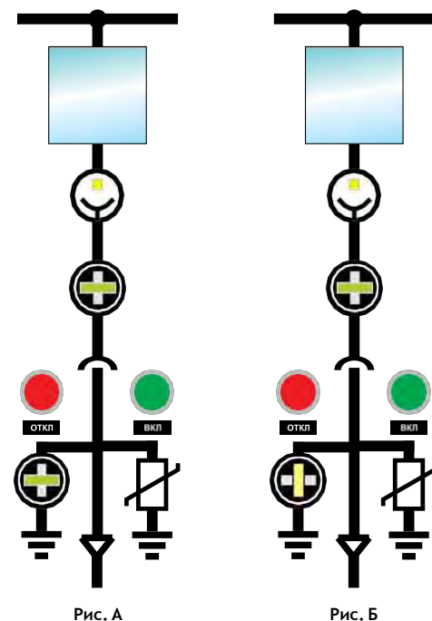
Рис. 1.48. Состояние мнемосхемы при нахождении КВЭ в контрольном положении
