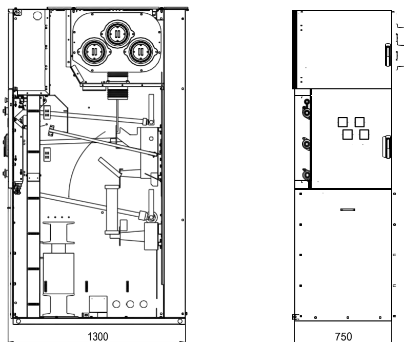
Рис. ПЗ.8. Шкаф КРУ D-12P с трансформатором собственных нужд до 40 кВа
