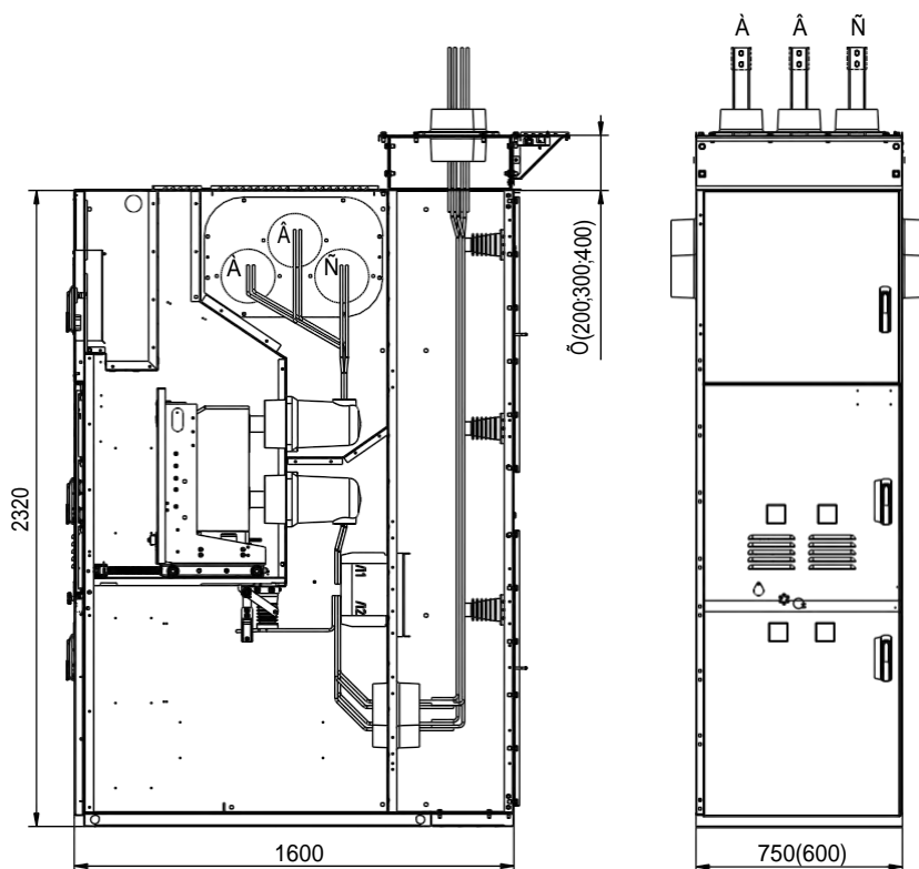
Рис. ПЗ.2. Шкаф КРУ D-12P с шинным вводом через заднюю приставку на номинальный ток до 2000 А
