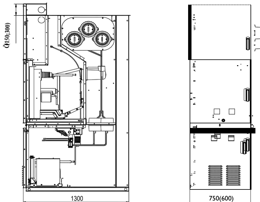
Рис. ПЗ.7. Шкаф КРУ D-12P с измерительными ТН
