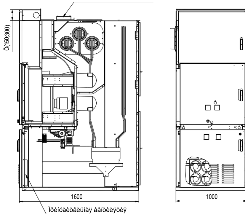
Рис. ПЗ.11. Шкаф КРУ D-12P с силовым выключателем на номинальный ток до 3150/4000 А и принудительной вентиляцией
