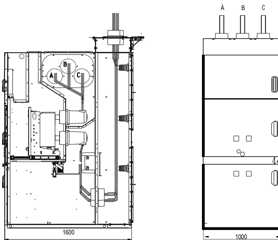
Рис. ПЗ.4. Шкаф КРУ D-12P с шинным вводом через заднюю приставку на номинальный ток до 3150 А
