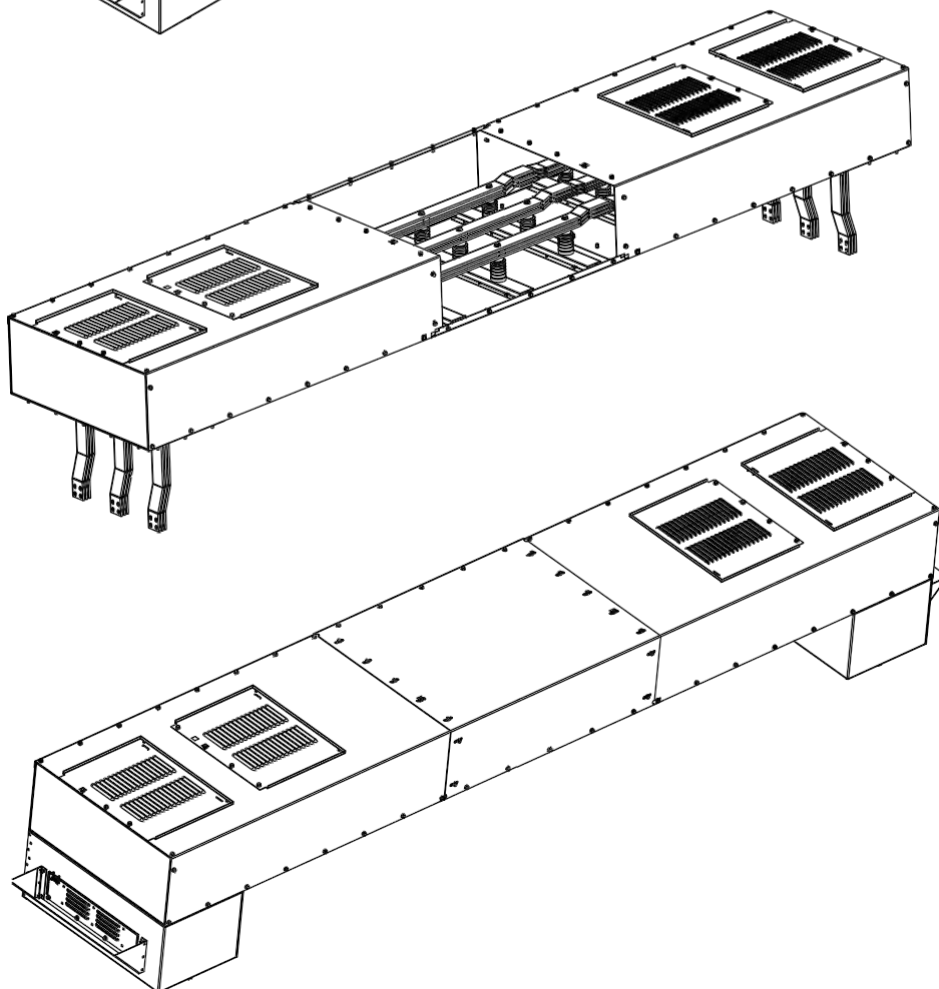
Рис. П7.7 Шинный мост в сборе
