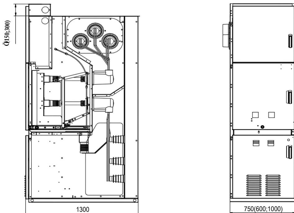
Рис. ПЗ.6 Шкаф КРУ D-12P с секционным разъединителем
