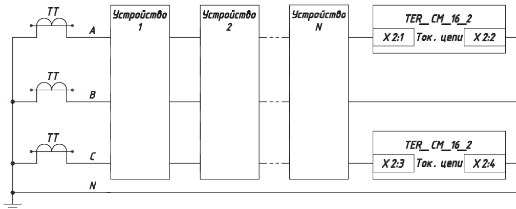
Рис.3.1. Подключение в цепь трансформаторов тока. Прямое включение
