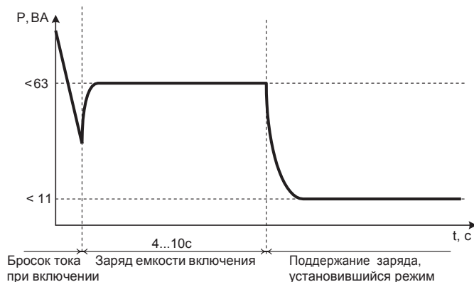
Рис.3.4. График потребления TER_CM_16_Type(220_Par2) при питании от переменного оперативного тока
