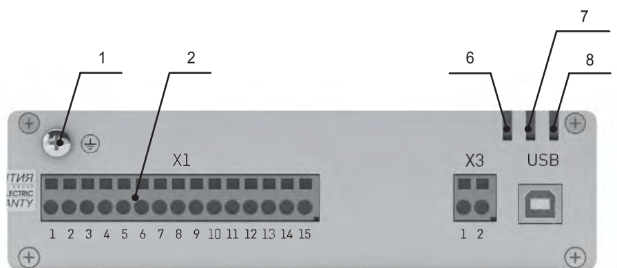
Модуль управления TER_CM_16_1
