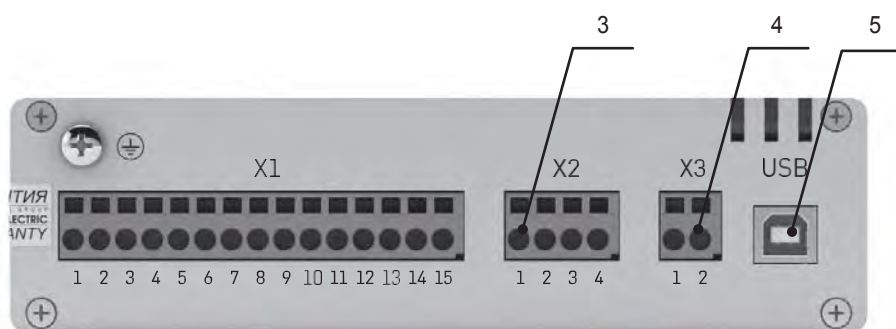
Модуль управления TER_CM_16_2, TER_CM_16_2D и TER_CM_16_FT
